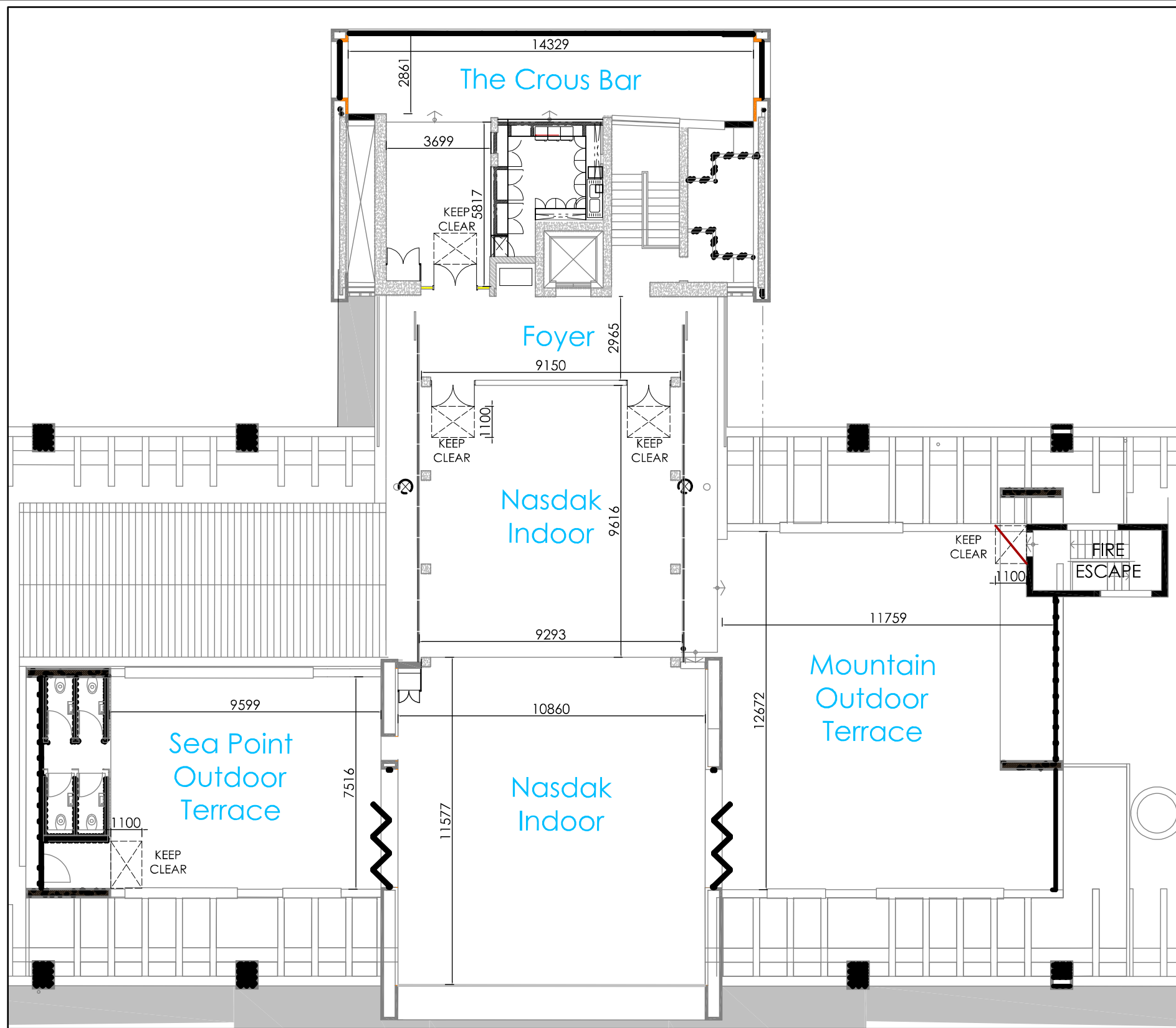
PLAN 26TH FLOOR (N.T.S)
